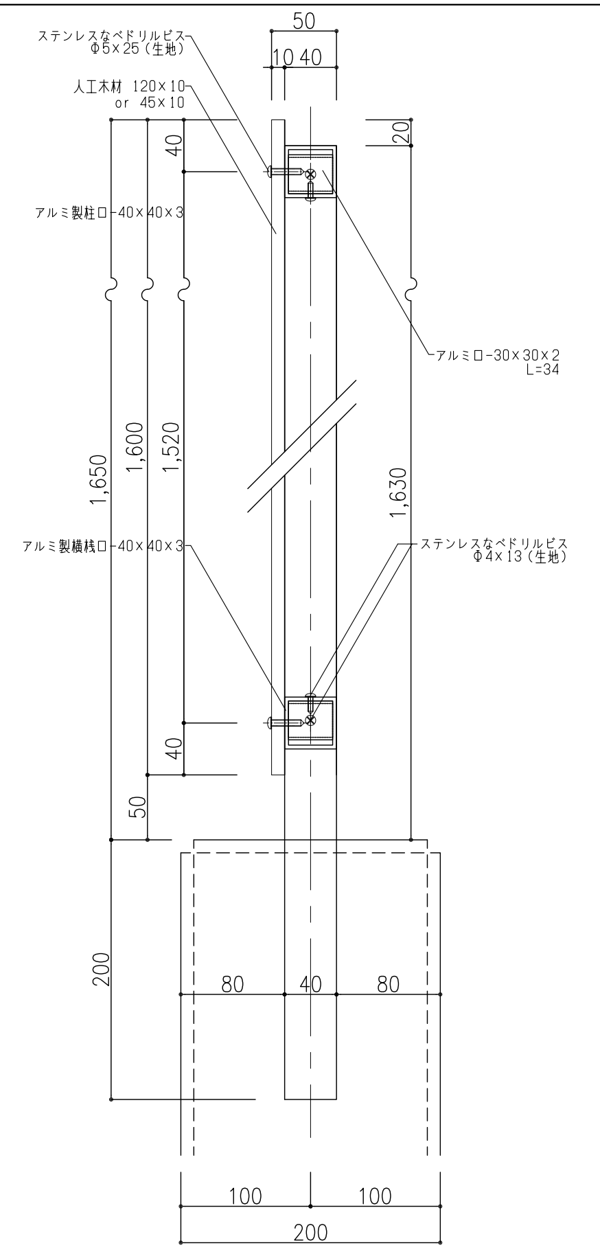
断面詳細図 S=1/4
